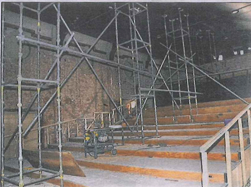
Speciale torenconstructies in de gestripte grote bioscoopzaal ondersteunen tijdelijk de bovenliggende verdiepingen.
